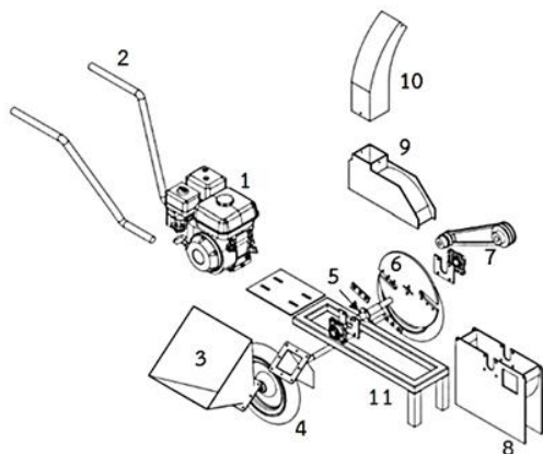
รูปที่ 5 ส่วนประกอบของเครื่องย่อยกิ่งไม้
