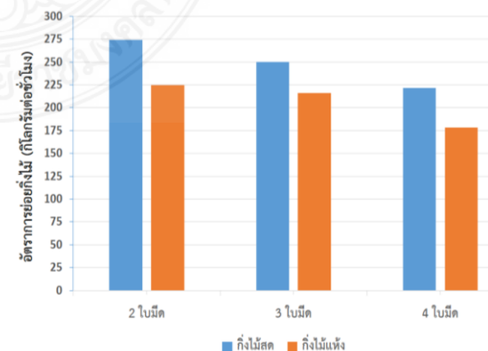
รูปที่ 8 อัตราการย่อยกิ่งไม้ (กิโลกรัมต่อชั่วโมง)
