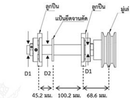
รูปที่ 3 การส่งกำลังเครื่องยนต์ผ่านสายพาน
