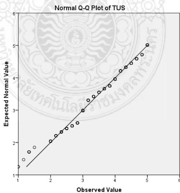
ภาพ 4.3 การแจกแจงของข้อมูลตัวแปรความไว้วางใจ (TUS)
