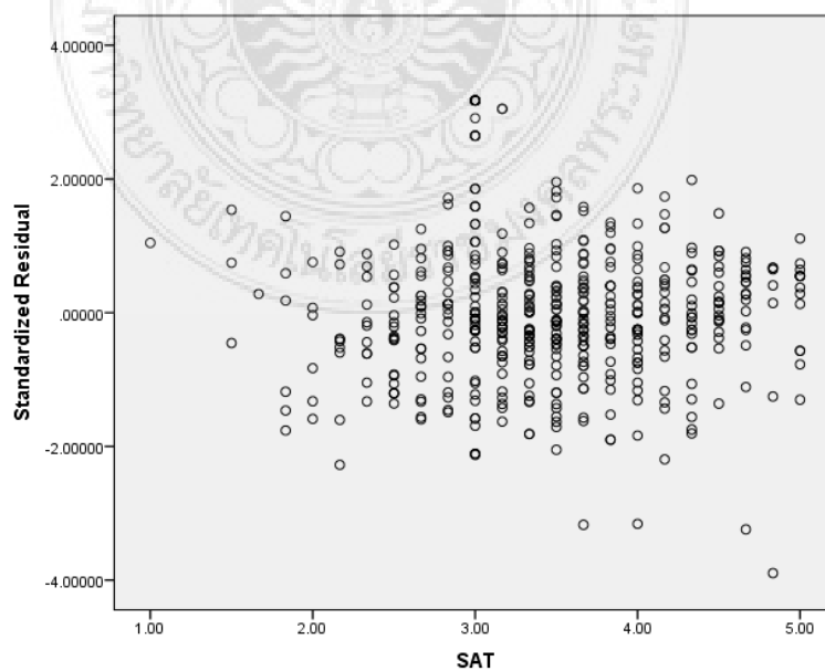
ภาพ 4.19 ความสัมพันธ์ระหว่างเศษที่เหลือ (Standardized Residual) กับตัวชี้วัดตัวแปรแฝง ความพึงพอใจของลูกค้า (SAT) ในกรณีที่มีการกลับมาใช้บริการซ้ำเป็นตัวแทน
