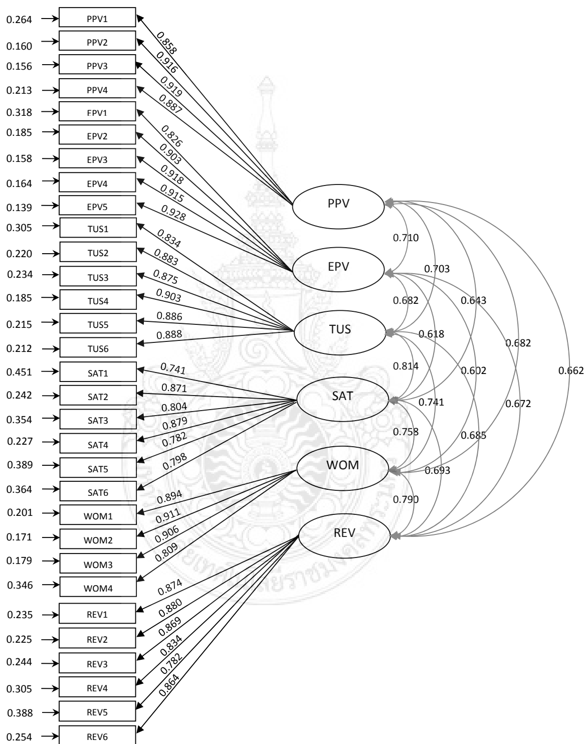
ภาพ 4.20 การวิเคราะห์หองค์ประกอบเชิงยืนยัน
