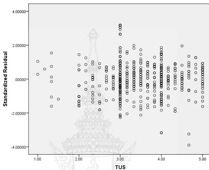
ภาพ 4.18 ความสัมพันธ์ระหว่างเศษที่เหลือ (Standardized Residual) กับตัวชี้วัดตัวแปรแฝง ความไวเนื้อเชื้อใจ (TUS) ในกรณีที่มีการกลับมาใช้บริการซ้ำเป็นตัวแทน
