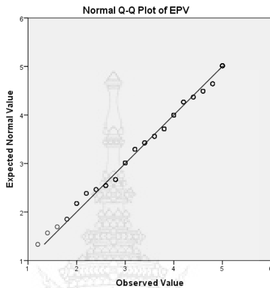
ภาพ 4.2 การแจกแจงของข้อมูลตัวแปรคุณค่าที่รับรู้ด้านอารมณ์ (EPV)
