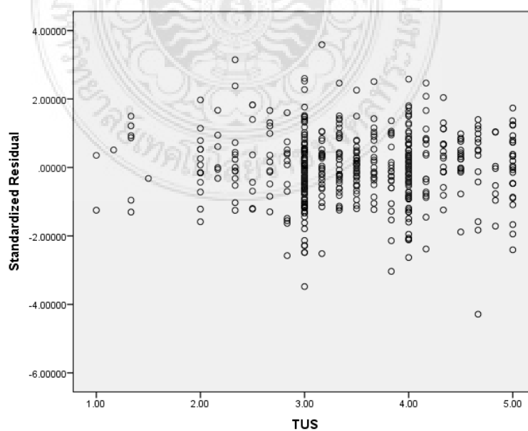
ภาพ 4.15 ความสัมพันธ์ระหว่างเศษที่เหลือ (Standardized Residual) กับตัวชี้วัดตัวแปรแฝง ความไว้วางใจ (TUS) ในกรณีที่ความพึงพอใจของลูกค้าเป็นตัวแปรตาม
