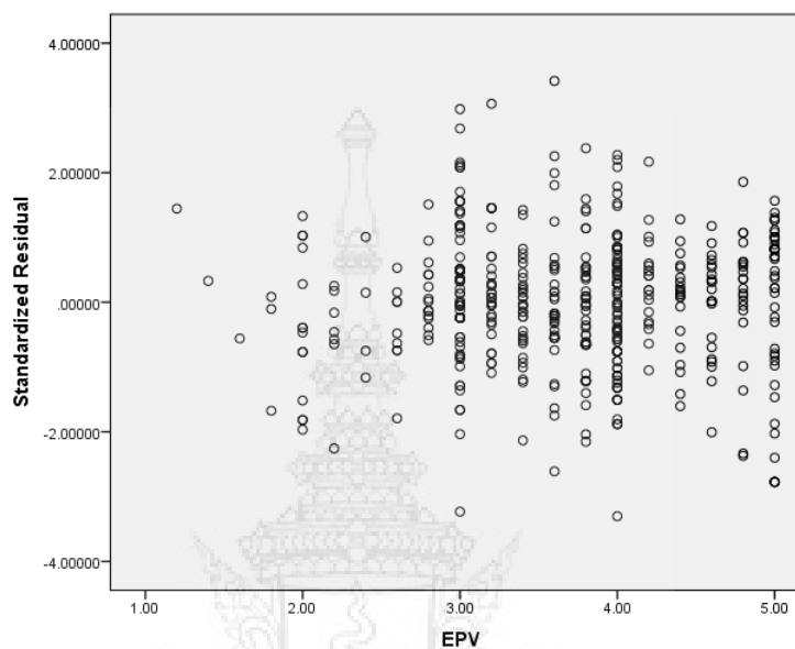
ภาพ 4.12 ความสัมพันธ์ระหว่างเศษที่เหลือ (Standardized Residual) กับตัวชี้วัดตัวแปรแฝง คุณค่าที่รับรู้ด้านอารมณ์ (EPV) ในกรณีที่ความไวเนื้อเชื้อใจ เป็นตัวแปรตาม
