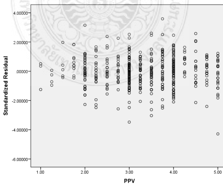
ภาพ 4.13 ความสัมพันธ์ระหว่างเศษที่เหลือ (Standardized Residual) กับตัวชี้วัดตัวแปรแฝง คุณค่าที่รับรู้ด้านราคา (PPV) ในกรณีที่ความพึงพอใจของลูกค้าเป็นตัวแปรตาม
