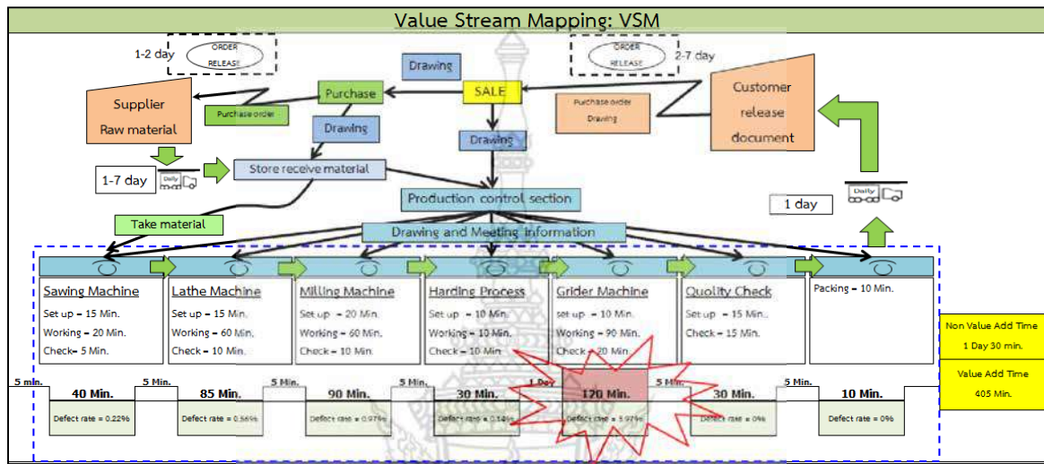
ภาพที่ 4 แผนภูมิสายธารแห่งคุณค่า (Value Stream Mapping: VSM) ก่อนการปรับปรุง
