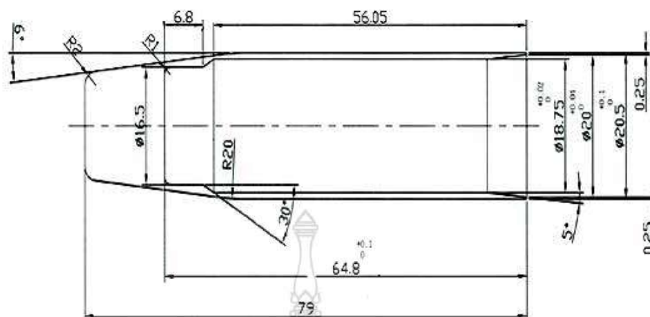
ภาพ 4.6 ตัวอย่าง ชิ้นงานชื่อ Protector (Job no.03-014)
