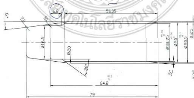
ภาพที่ 10 ตัวอย่าง ชิ้นงานชื่อ Protector (Job no.03-014)
