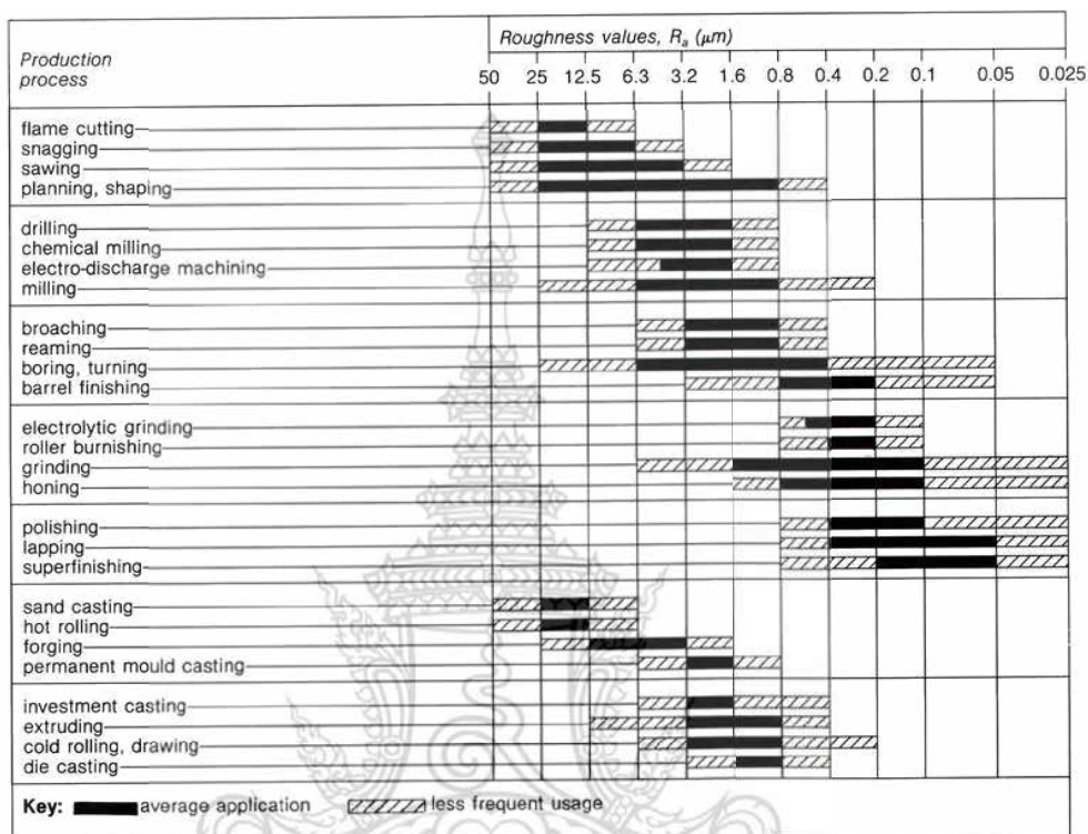
ภาพ 2.3 ความหยาบของผิวงานกับกระบวนการผลิต ที่มา: บรรเลง (2549)
