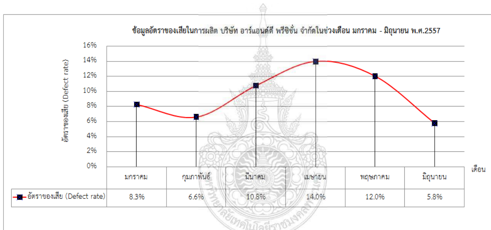
ภาพ 3.3 ข้อมูลอัตราของเสียการผลิตชิ้นงานความเที่ยงตรงสูงเดือนมกราคม ถึง มิถุนายน พ.ศ.2557 ที่มา: บริษัท อาร์แอนดีพี รีซิชัน จำกัด
