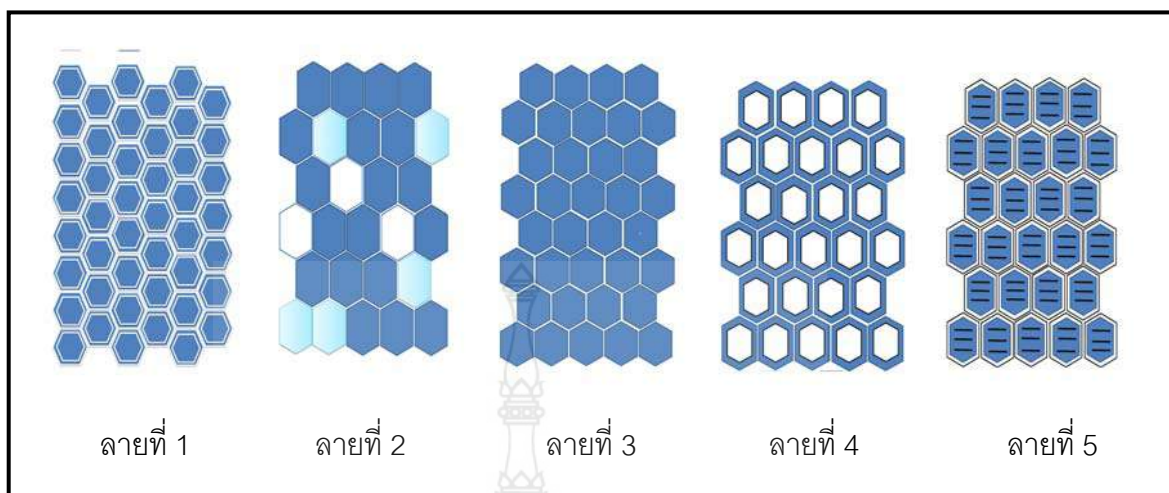
ภาพที่ 3.3 ลวดลายจากรูปหกเหลี่ยม
