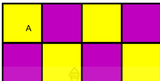
ภาพที่ 2.5 ลักษณะการเรียงภาพเทสเซลเลชันรูปสี่เหลี่ยม ที่มา: ศักดา (2548)
