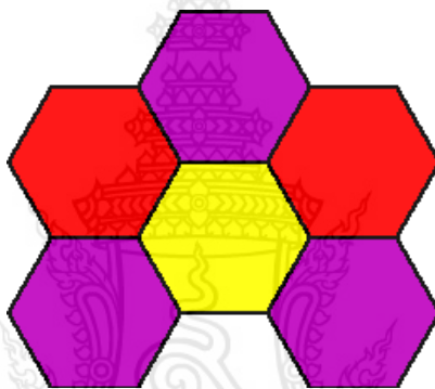
ภาพที่ 2.1 ลักษณะการเรียงภาพเทสเซลเลชันแบบปรกติ
