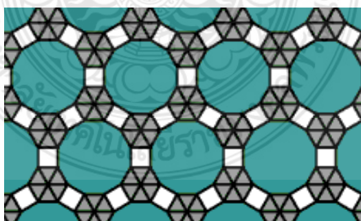
ภาพที่ 2.3 ลักษณะการเรียงภาพเทสเซลเลชันแบบเดมิเรกิวลาร์
