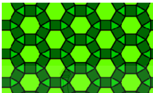
ภาพที่ 2.2 ลักษณะการเรียงภาพเทสเซลเลชันแบบกึ่งปกติ
