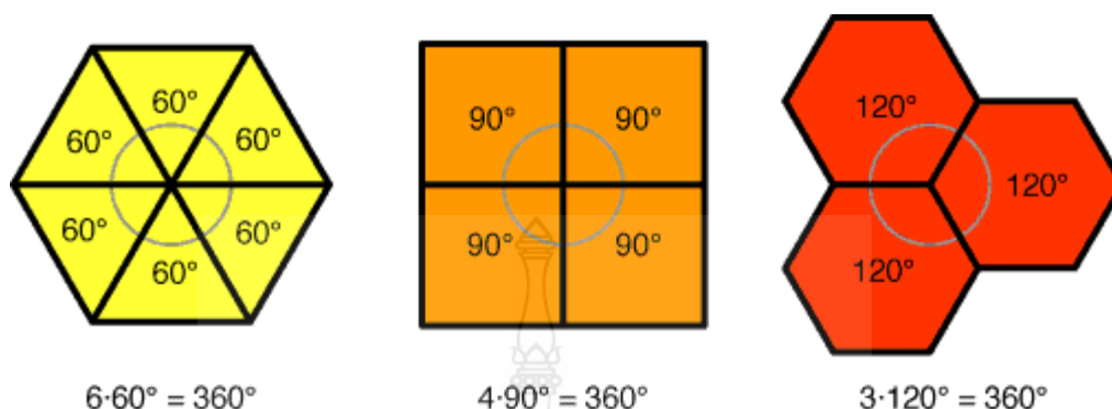
ภาพที่ 2.7 แสดงผลบวกของมุมที่จุดร่วมของรูปเหลี่ยมชนิดต่าง ๆ
