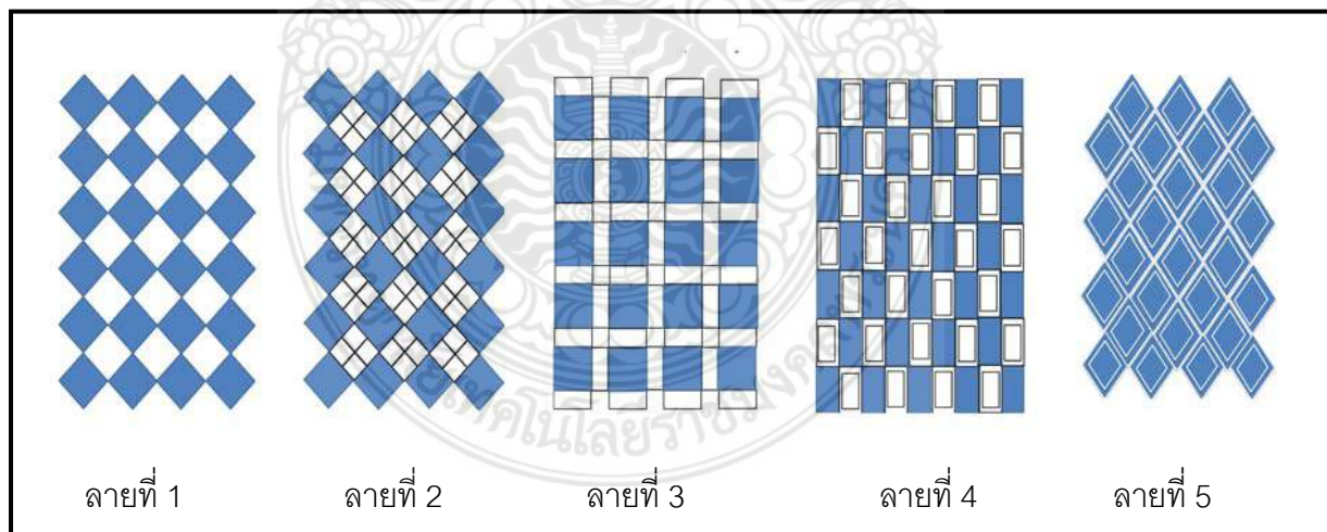
ภาพที่ 3.2 ลวดลายจากรูปสี่เหลี่ยม
