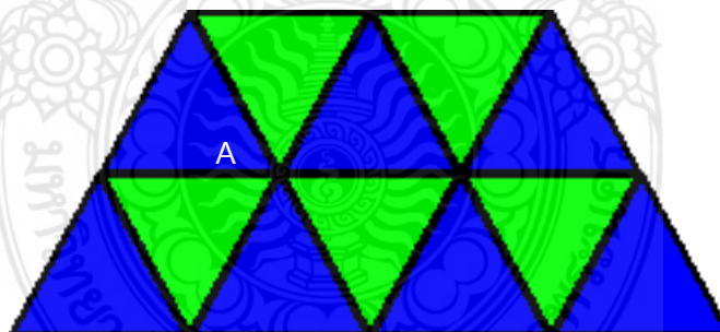
ภาพที่ 2.4 ลักษณะการเรียงภาพเทสเซลเลชันรูปสามเหลี่ยม ที่มา: ศักดา (2548)
