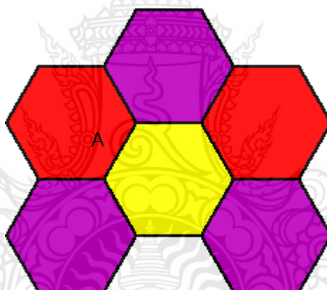
ภาพที่ 2.6 ลักษณะการเรียงภาพเทสเซลเลชันรูปหกเหลี่ยม ที่มา: ศักดา (2548)
