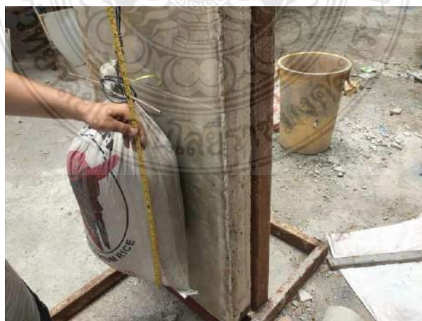
รูปที่ 8 การใช้วัสดุนุ่มขนาดใหญ่สำหรับทดสอบความทนต่อการกระแทกของแผ่นผนังคอนกรีตสำเร็จรูปมวลเบาเสริมแผ่นโฟมอัดแน่น
