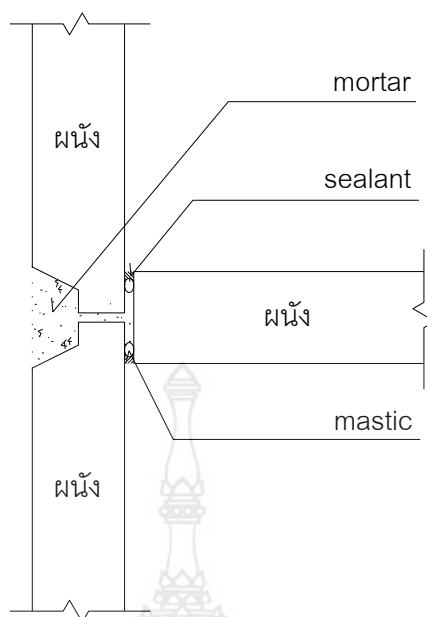
รูปที่ 2.34 แปลนรอยต่อผนังกับผนังริมนอกของอาคาร
