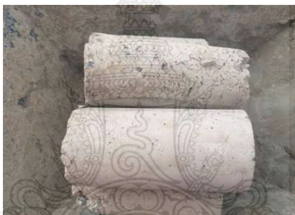
รูปที่ 3.40 แท่งมอร์ตาร์ทรงกระบอกที่วิบัติจากการทดสอบความต้านทานแรงอัด
