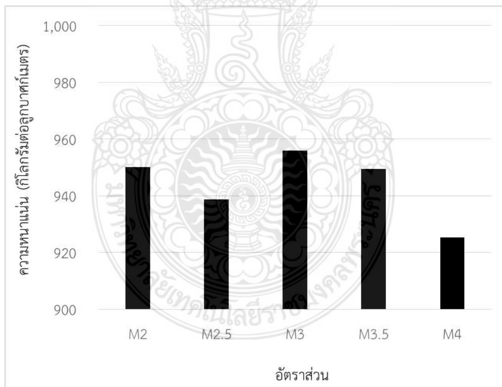
รูปที่ 14 ความหนาแน่นของผนังคอนกรีตมวลเบาด้วยการเสริมแผ่นโฟมอัดแน่น ที่อายุการบ่ม 28 วัน
