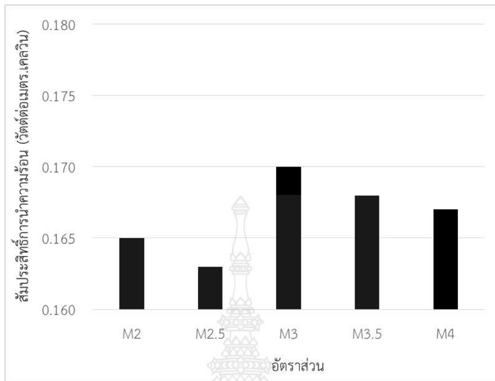
รูปที่ 16 สัมประสิทธิ์การนำความร้อนของผนังคอนกรีตมวลเบาด้วยการเสริมแผ่นโคมอัดแน่น ที่อายุการบ่ม 28 วัน
