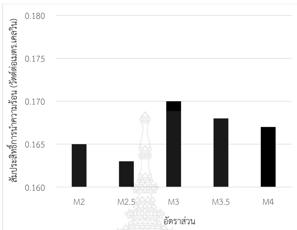
รูปที่ 4.15 สัมประสิทธิ์การนำความร้อนของผนังคอนกรีตมวลเบาด้วยการเสริมแผ่นโฟมอัดแน่น ที่อายุการบ่ม 28 วัน
