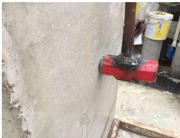
รูปที่ 3.13 ต้มน้ำหนักสำหรับแท่นทดสอบความทนการกระแทก
