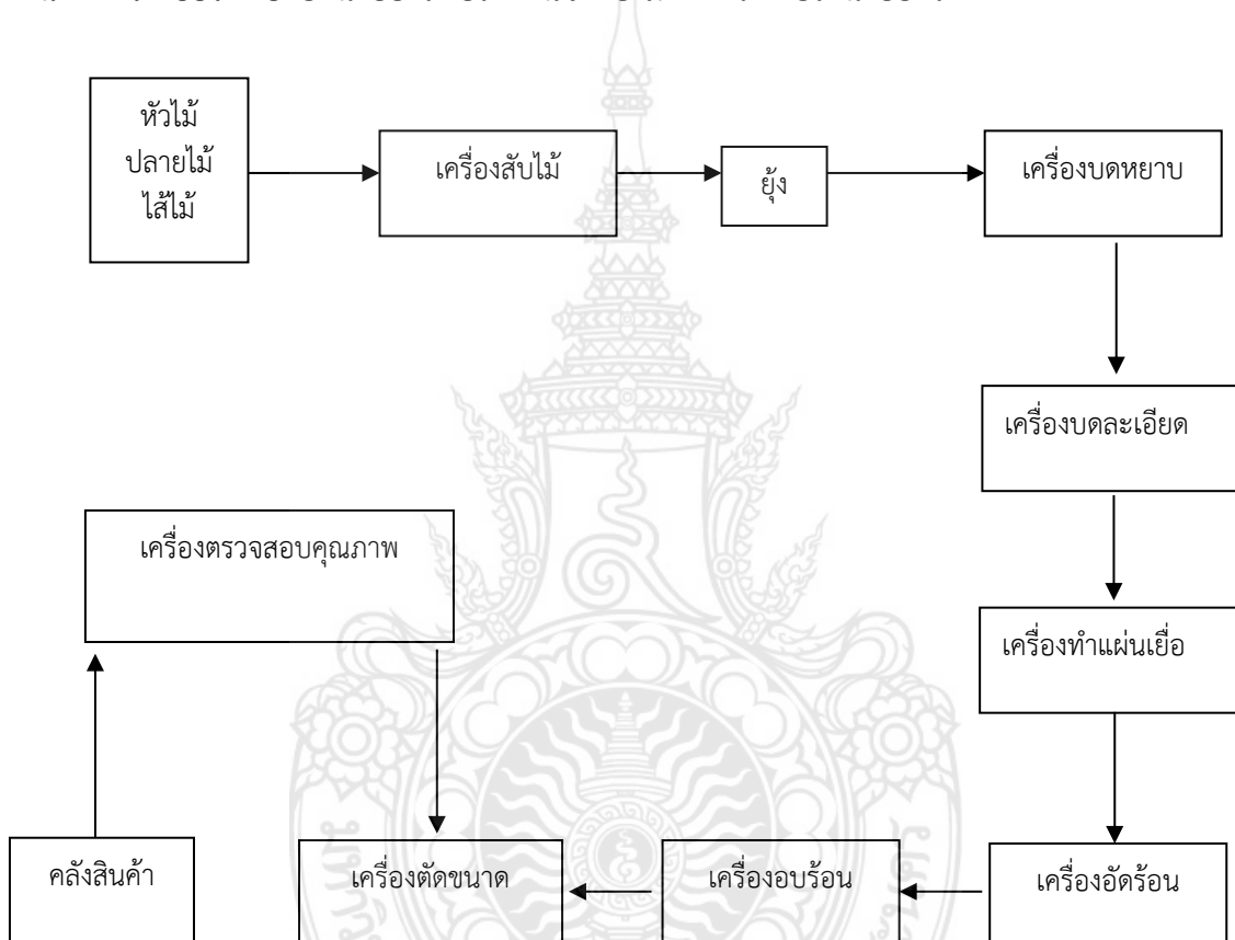
รูปที่ 2.2 กรรมวิธีการผลิตไม้อัดแผ่นเรียบวิธีที่ 1 (ณรงค์, 2517)
