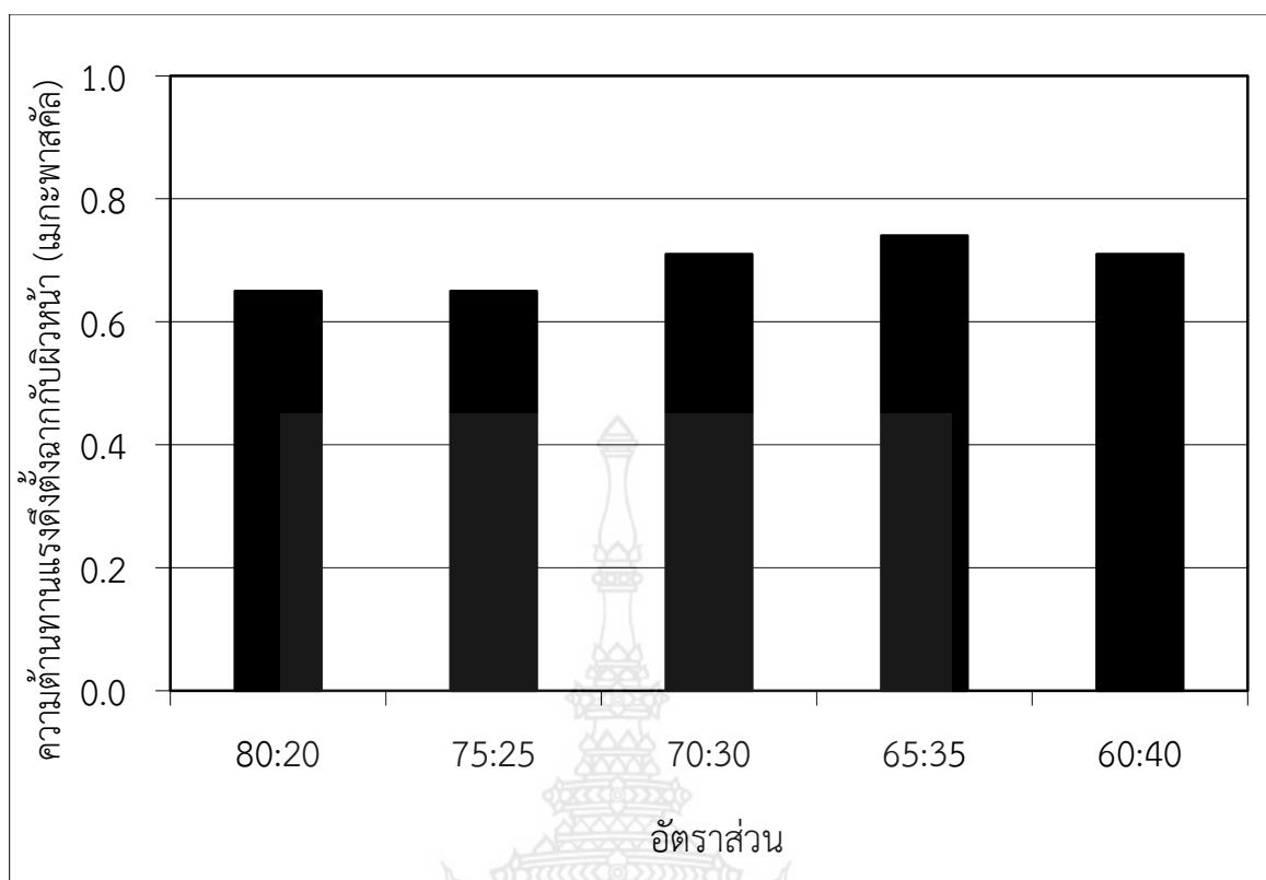
รูปที่ 4.11 ความต้านทานแรงดึงตั้งฉากกับผิวหน้าของแผ่นไม้เทียมจากขยะกล่องนมผสมเศษพลาสติก PET อัตราส่วนต่างๆ
