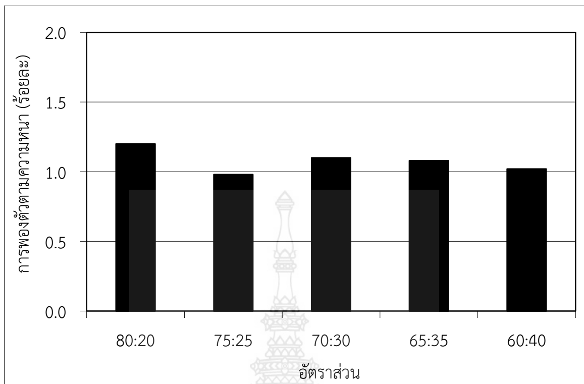
รูปที่ 4.8 การพองตัวตามความหนาของแผ่นไม้เทียมจากขยะกล่องนมผสมเศษพลาสติก PET อัตราส่วนต่างๆ
