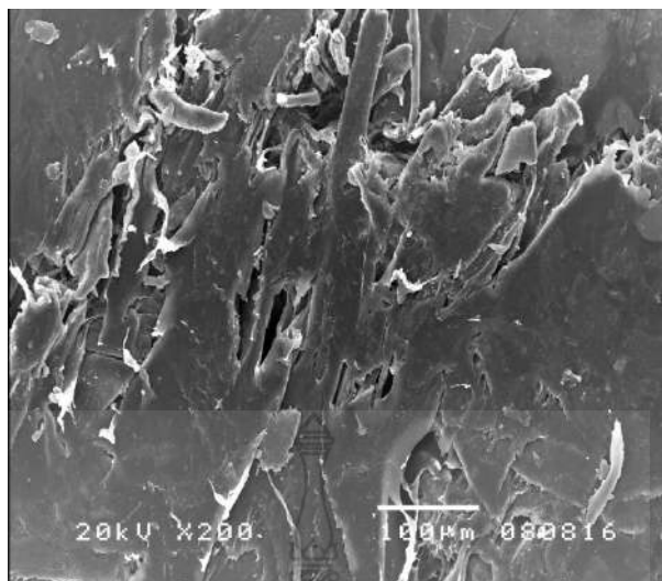
รูปที่ 4.14 ผิวหน้าของแผ่นไม้เทียมจากเศษกระดาษกล่อนผสมพลาสติก PET จากกล้อง SEM ที่กำลังขยาย 200 เท่า
