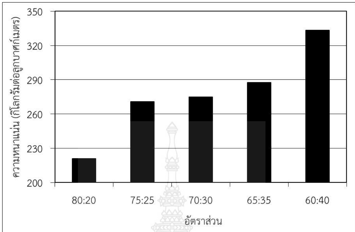
รูปที่ 20 ความหนาแน่นของแผ่นไม้เทียมจากขยะกล่องนมผสมเศษพลาสติก PET อัตราส่วนต่างๆ
