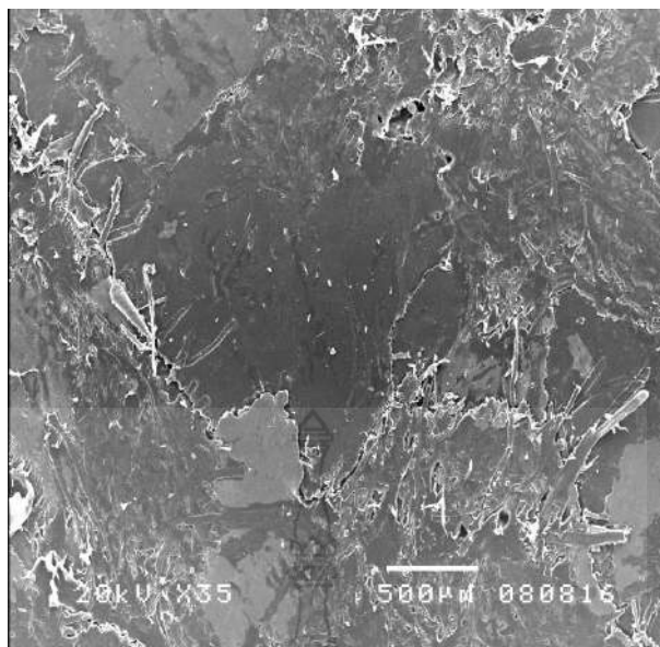
รูปที่ 4.12 ผิวหน้าของแผ่นไม้เทียมจากเศษกระดาษกล่อนมผสมเศษพลาสติก PET จากกล้อง SEM ที่กำลังขยาย 35 เท่า
