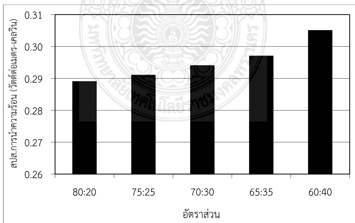
รูปที่ 4.15 สัมประสิทธิ์การนำความร้อนของแผ่นไม้เทียมจากขยะกล่อนผสมพลาสติก PET อัตราส่วนต่างๆ
