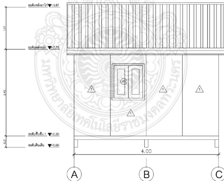
รูปที่ 5 แบบด้านซ้ายของบ้านถอดประกอบที่ชนส่งสะดวกเพื่อผู้ประสบภัย
