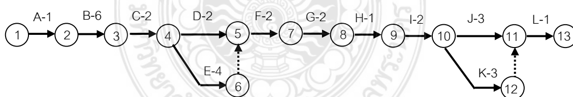
รูปที่ 4.6 แผนการก่อสร้างบ้านถอดประกอบที่ขนส่งสะดวกเพื่อผู้ประสบภัยด้วยวิธี CPM (Critical Path Method)
