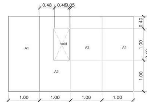
A แบบขยายผนังภายนอก F-01-1 1:50
