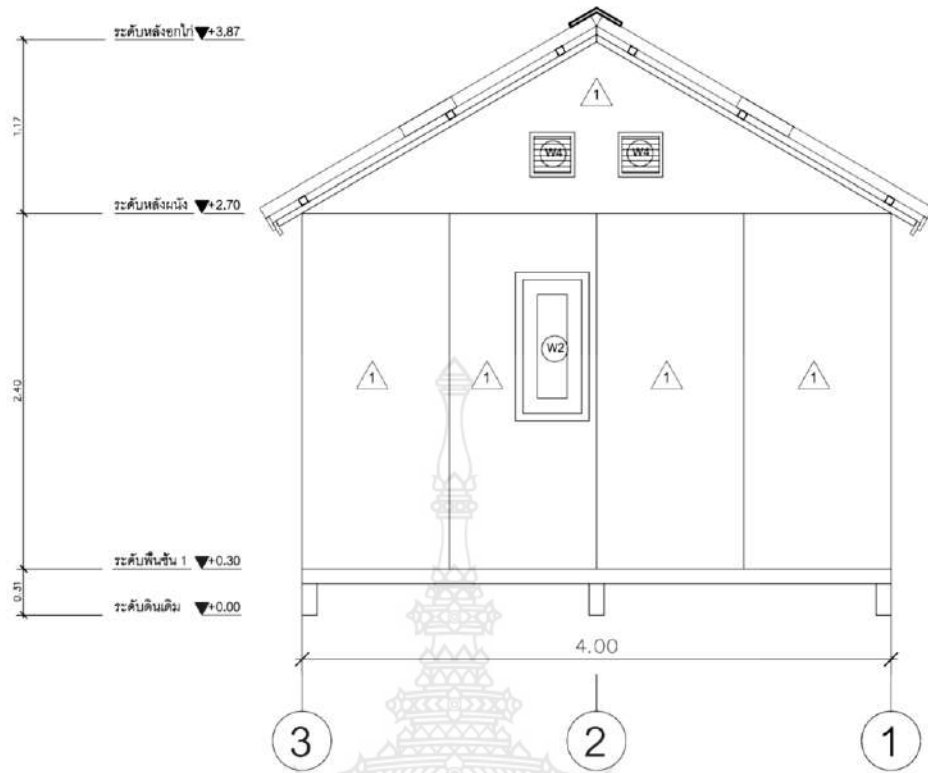
รูปที่ 4 แบบด้านหลังของบ้านถอดประกอบที่ชนส่งสะดวกเพื่อผู้ประสบภัย
