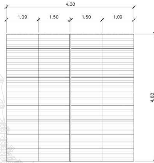
แปลนหลังคา 1 : 50
