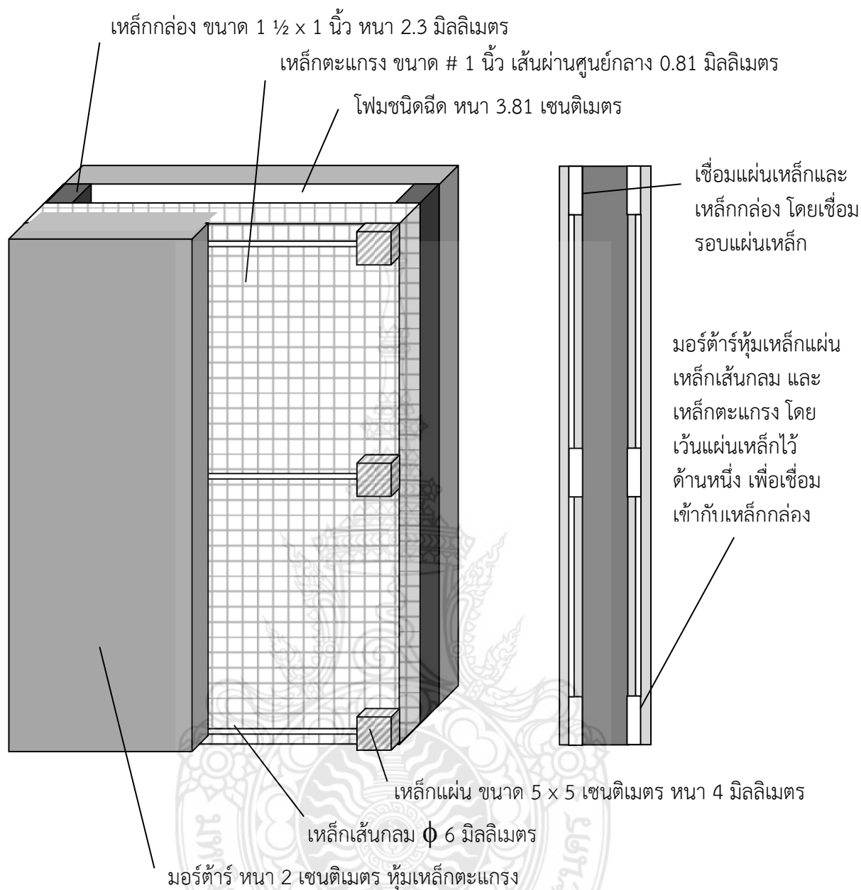
รูปที่ 3.13 ส่วนประกอบของผนังคอนกรีตสำเร็จรูปมวลเบาด้วยเทคนิคการฉีกโฟมเป็นแกนกลางผนัง
