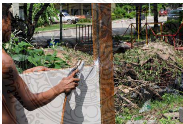
รูปที่ 4.15 การเชื่อมผนังคอนกรีตสำเร็จรูปมวลเบาด้วยวิธีฉีดโฟมเป็นแกนกลางเข้ากับเสาเหล็กโดยใช้ลวดเชื่อมไฟฟ้า
