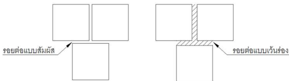
รูปที่ 2.4 รอยต่อแบบสัมผัสและแบบเว้นร่อง
