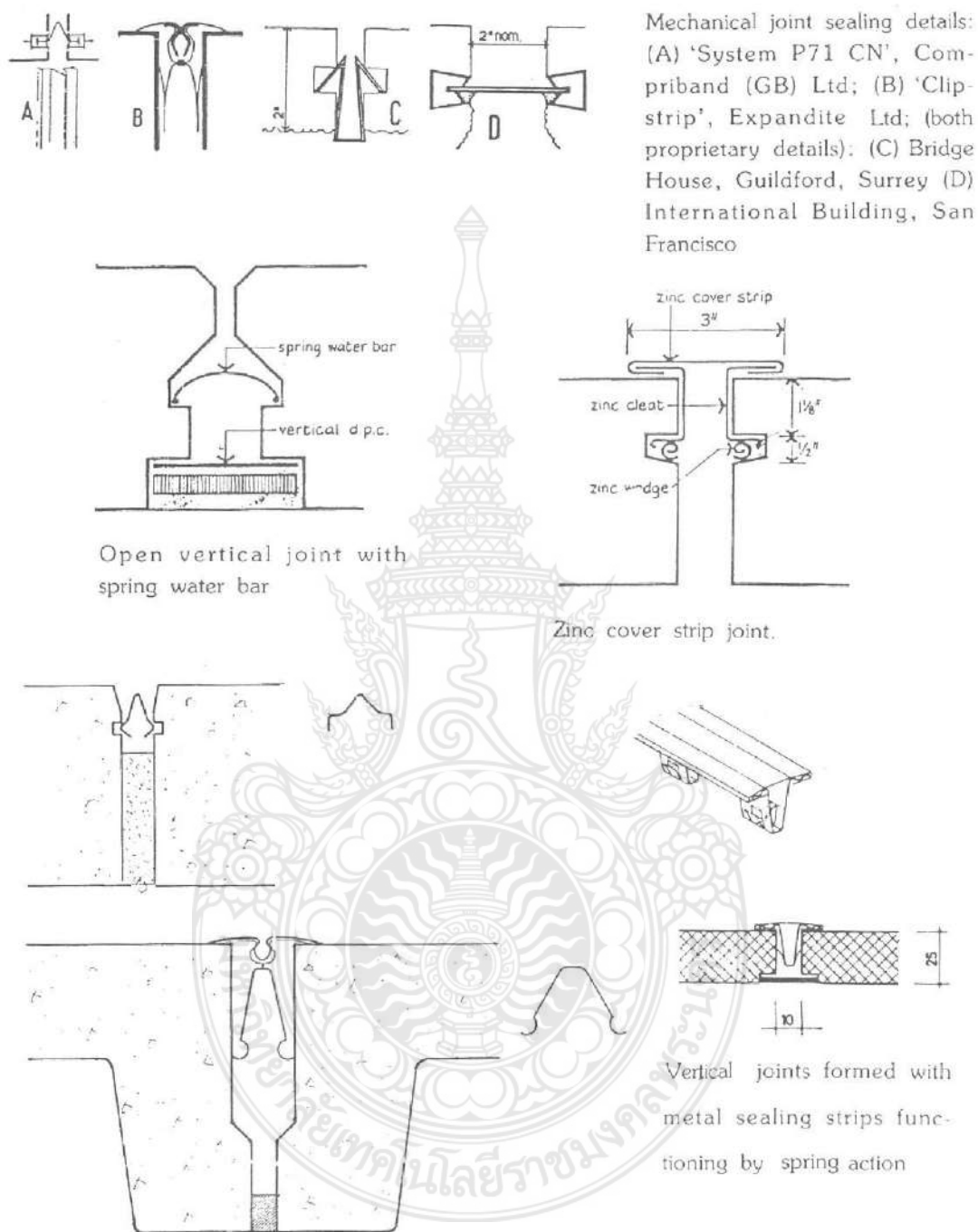
รูปที่ 2.23 ตัวอย่างรอยต่อแบบกลไก (Mechanically- Sealed Joints)
