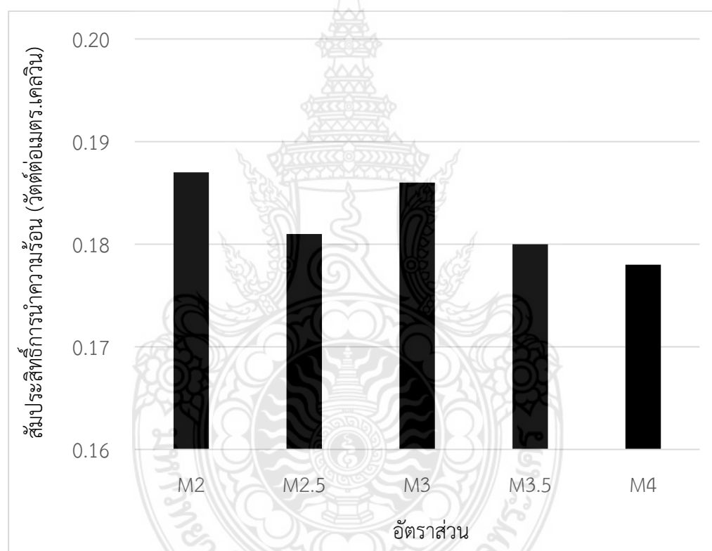
รูปที่ 4.13 สัมประสิทธิ์การนำความร้อนของผนังคอนกรีตสำเร็จรูปมวลเบาด้วยวิธีฉีดยาเป็นแกนกลาง ที่อายุการบ่ม 28 วัน
