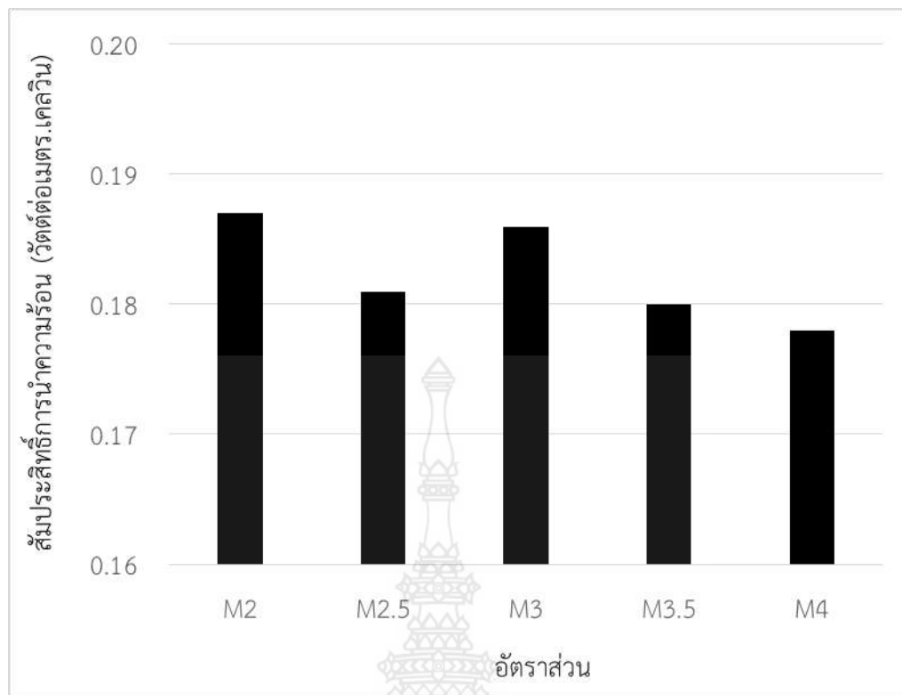
รูปที่ 19 สัมประสิทธิ์การนำความร้อนของผนังคอนกรีตสำเร็จรูปมวลเบาด้วยวิธีฉีดโฟมเป็นแกนกลาง ที่อายุการบ่ม 28 วัน
