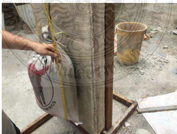
รูปที่ 3.55 การยกวัสดุหนุนให้ได้มุมและระดับตามที่มาตรฐานกำหนด
