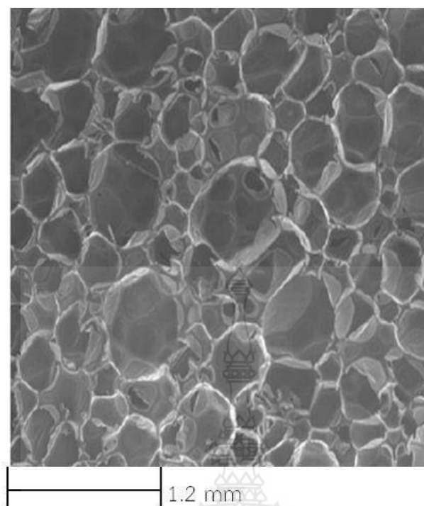
รูปที่ 3.12 อณูฐานของโฟมชนิดฉีดยาจากกล้องจุลทรรศน์อิเล็กตรอนแบบส่องกราด (SEM) ที่กำลังขยาย 50 เท่า
