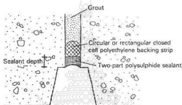
รูปที่ 2.16 ตัวอย่างการใช้ Polyethylene กำหนดความหนาของวัสดุยาแนว
