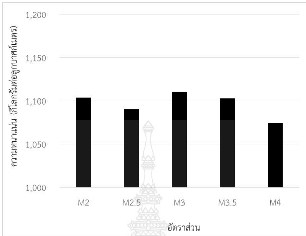
รูปที่ 17 ความหนาแน่นของผืนคอนกรีตสำเร็จรูปมวลเบาด้วยวิธีฉีดโฟมเป็นแกนกลาง ที่อายุการบ่ม 28 วัน
