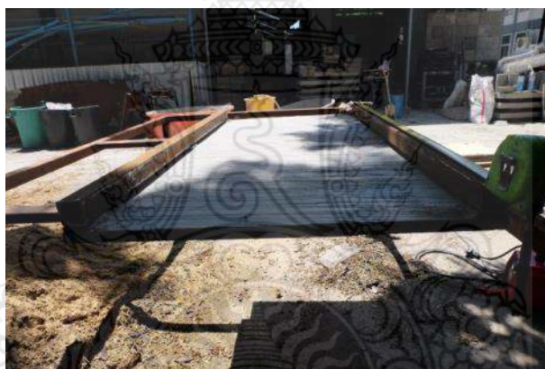
รูปที่ 3.27 การเตรียมการติดตั้งแผ่นมอร์ตาร์สำหรับเป็นผนังสำเร็จรูป
