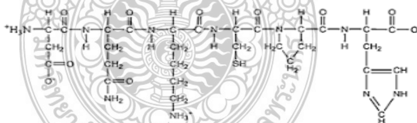
ภาพที่ 2.3 ลักษณะโครงสร้างของเอนไซม์
