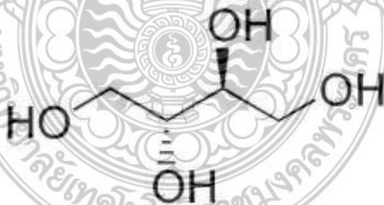
ภาพที่ 2.14 ลักษณะโครงสร้างอิริไซโทล
