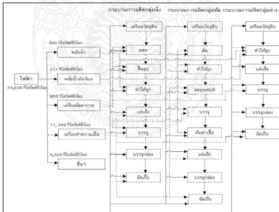
ภาพ 4.8 ผังสมดุลมวลการใช้ไฟฟ้าต่อวัน
