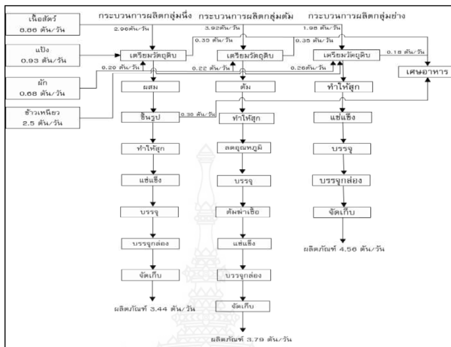
ภาพ 4.5 ฟังสมดุลงานการผลิต
