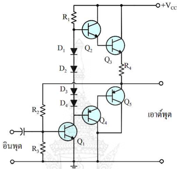
ภาพที่ 2.34 วงจรถวายสัญญาณเสียงแบบดาร์lington [8]
