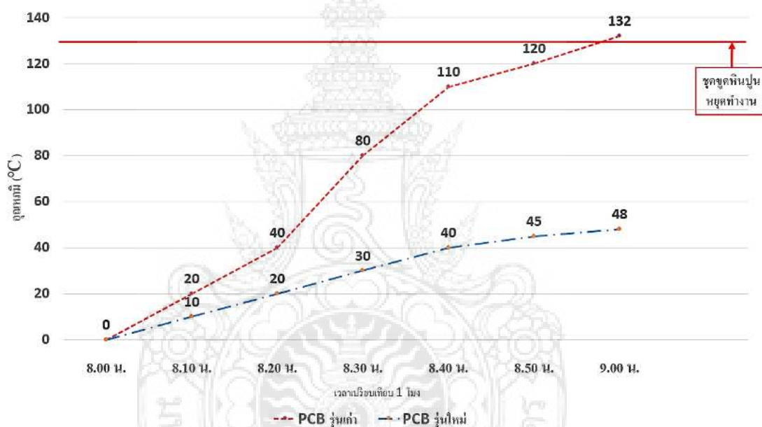
ภาพที่ 4.14 กราฟแสดงการทดสอบเปรียบเทียบอุณหภูมิวงจรขยายสัญญาณทำงานต่อเนื่อง 1 ชั่วโมง
