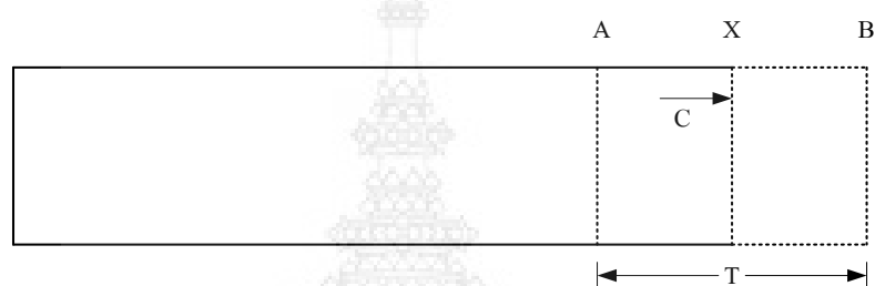
ภาพที่ 2.8 การเคลื่อนที่ของแท่งทรานสดิวเซอร์ในสนามไฟฟ้า [3]
