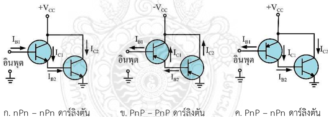
ภาพที่ 2.33 ทรานซิสเตอร์แบบดาร์ลิงตัน [8]
