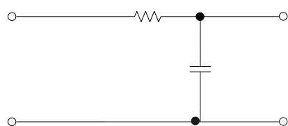
(a) วงจรอันดับ 1
