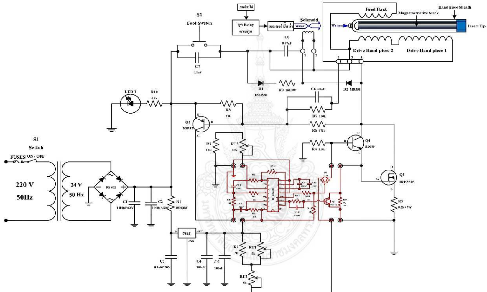
ภาพที่ ข-2 วงจรภาพรวมของเครื่องชุดหินปูนแบบอัลตราโซนิก (ULTaSONIC SCaLEr)
