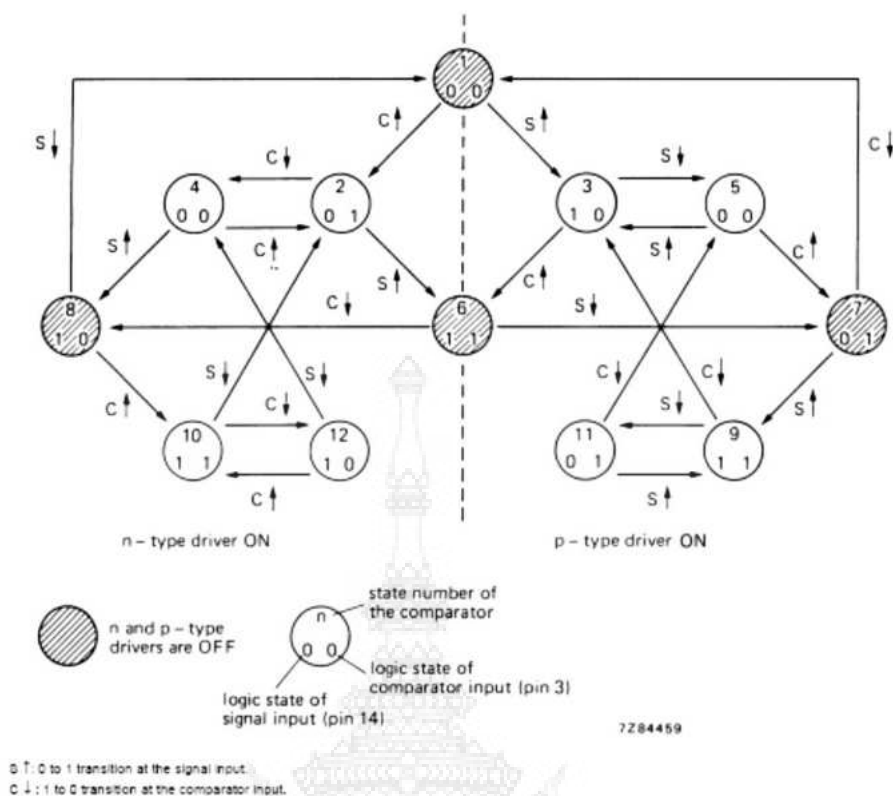
ภาพที่ 3.9 การเปลี่ยนแปลงลอจิกที่สัญญาณอินพุต (S) หรืออินพุต (c) เปรียบเทียบการเปลี่ยนแปลงขอบขาขึ้นและขอบขาลง แสดงด้วยลูกศรชี้ขึ้นหรือลงตามลำดับ [9]
