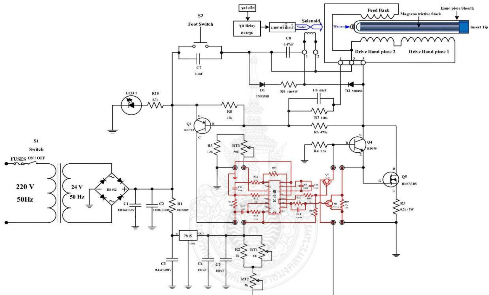
ภาพที่ 3.3 วงจรภาพรวมของเครื่องชุดหินปูนแบบอัลตราโซนิค (Ultrasonic scalar)
