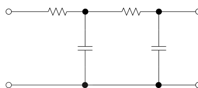
(b) วงจรอันดับ 2
