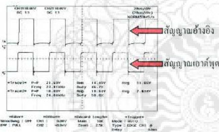
รูปที่ 9 สัญญาณที่ออกจากร่างวงจรชุดหัวชุดหุนปืนหลังปรับปรุง
