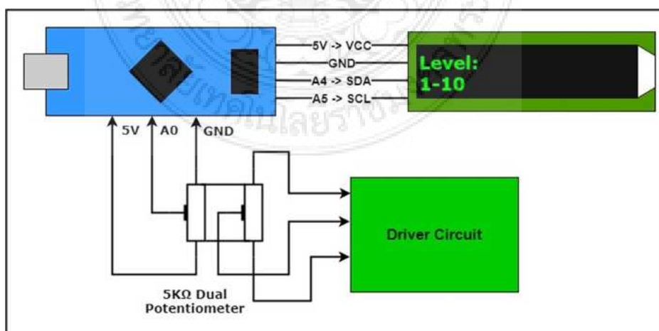
ภาพที่ 3.11 วงจรจอแสดงผลการปรับระดับด้วย arduino nano
