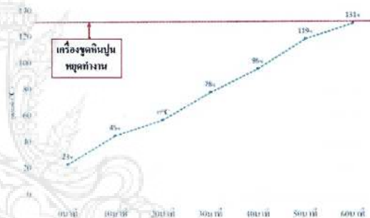
รูปที่ 6 อุณหภูมิทรานซิสเตอร์ตำแหน่งที่ 2 ของวงจรขยายสัญญาณ
