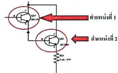
รูปที่ 5 ตำแหน่งความร้อนที่เกิดขึ้นกับทรานซิสเตอร์ทั้งสองตัว
