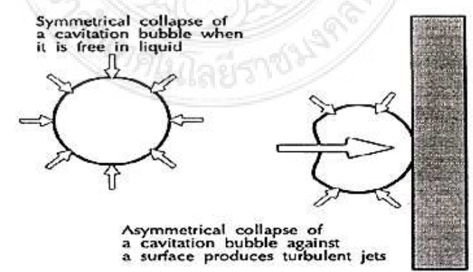
ภาพที่ 2.20 Energy jets by ultrasonic ca-itation [3]
