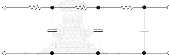
(c) วงจรอันดับ 3
