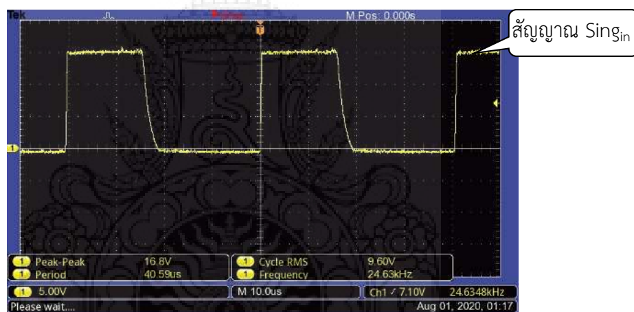
ภาพที่ 4.6 สัญญาณวัดที่ขา 14 ( S_{in} ) ของไอซีเบอร์ 4046b เทียบกับขา 8 ( V_{ss} )
