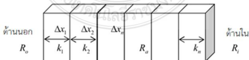
รูปที่ 2.2 ค่าความต้านทานความร้อนจากวัสดุต่างชนิดกันและมีช่องว่างอากาศภายใน
