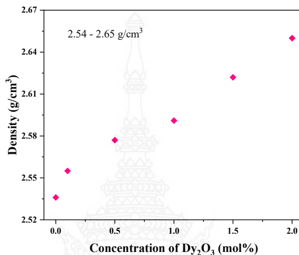
ภาพที่ 4.2 กราฟแสดงความสัมพันธ์ระหว่างความหนาแน่นของแก้วตัวอย่างกับปริมาณความเข้มข้นของ Dy_2O_3
