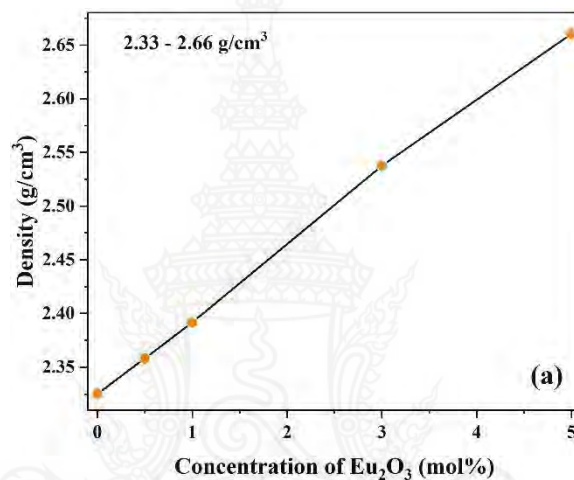
ภาพที่ 4.18 กราฟแสดงความสัมพันธ์ระหว่างความหนาแน่นของแก้วตัวอย่างกับปริมาณความเข้มข้นของ \text{Eu}_2\text{O}_3
