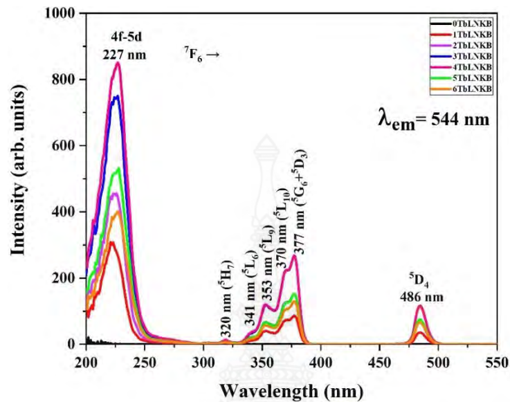
ภาพที่ 4.12 สเปกตรัมการกระตุ้นแสงของแก้วตัวอย่าง LNKB ที่เจือด้วย Tb_2O_3 ที่ความเข้มข้นต่าง ๆ
