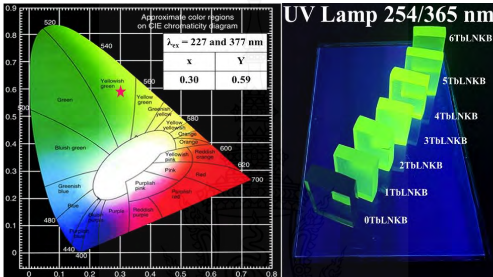
ภาพที่ 4.15 สีของการเปล่งแสงในระบบ CIE 1931 ของ Tb^{3+} เติมในแก้ว LNKB
