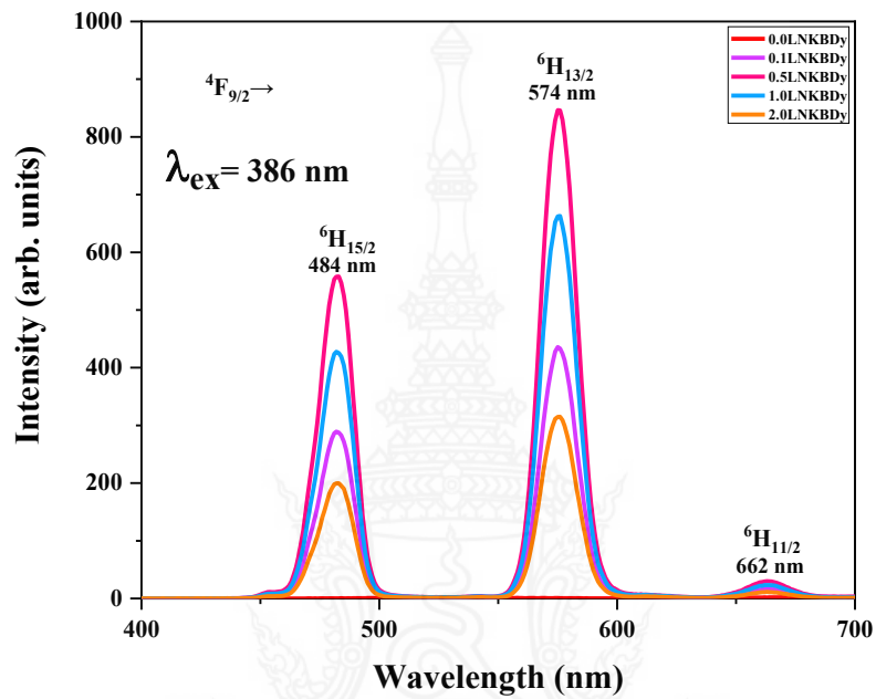
ภาพที่ 4.6 สเปกตรัมการเปล่งแสงจากการกระตุ้นด้วยแสงของแก้วตัวอย่าง LNKB ที่เจือด้วย Dy_2O_3 ที่ความเข้มข้นต่าง ๆ
