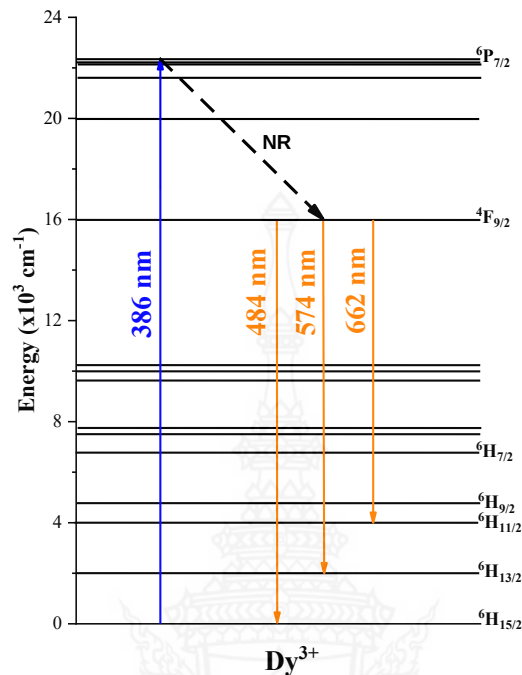
ภาพที่ 4.7 การเปลี่ยนแปลงระดับชั้นพลังงานของ \text{Dy}^{3+} เต็มในแก้ว LNKB ตามสเปกตรัมการเปล่งแสง
