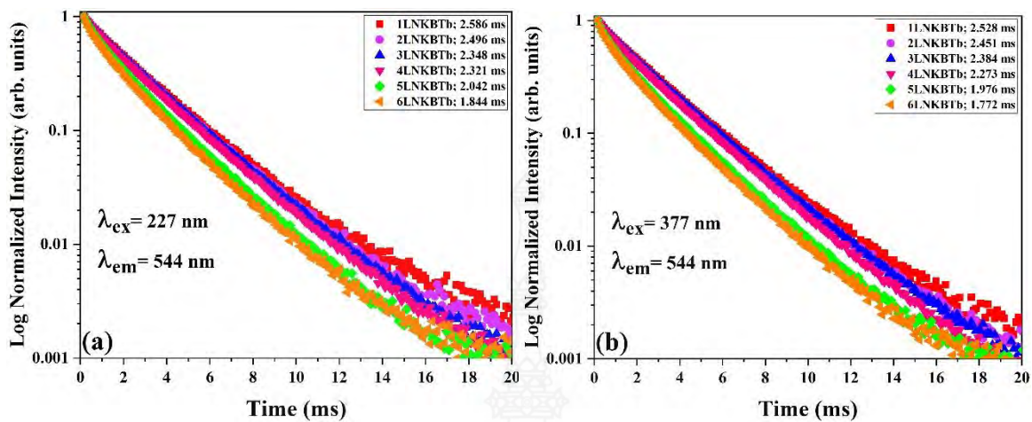
ภาพที่ 4.16 เวลาการสลายตัวของ Tb^{3+} เติมในแก้ว LNKB
