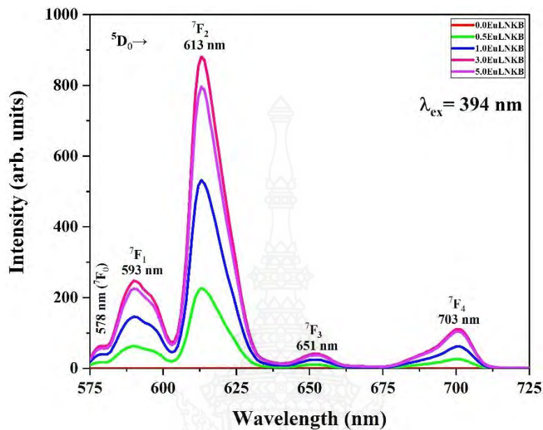
ภาพที่ 4.22 สเปกตรัมการเปล่งแสงของแก้วตัวอย่าง LNKB ที่เจือด้วย \text{Eu}_2\text{O}_3 ที่ความเข้มข้นต่าง ๆ
