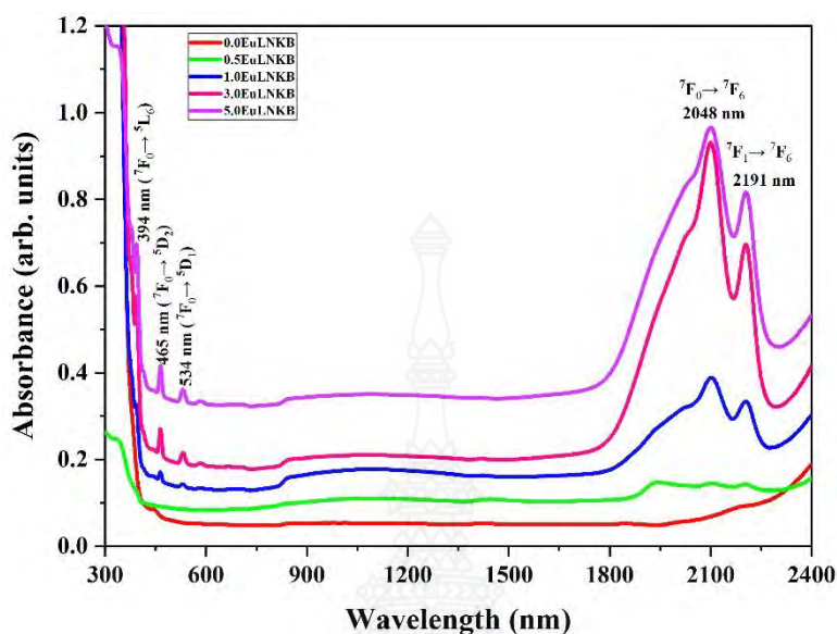
ภาพที่ 4.20 สเปกตรัมการดูดกลืนแสงของแก้วตัวอย่าง LNKb ที่เจือด้วย \text{Eu}_2\text{O}_3 ที่ความเข้มข้นต่าง ๆ
