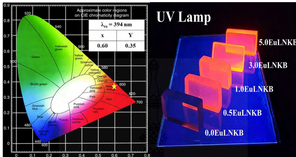
ภาพที่ 4.23 สีของการเปล่งแสงในระบบ CIE 1931 ของ \text{Eu}^{3+} เติมในแก้ว LNKB
