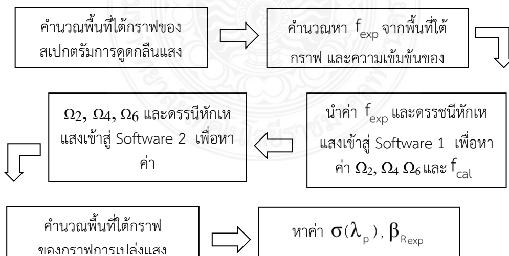
ภาพที่ 3.8 แผนผังการวิเคราะห์ Judd-Ofelt (JO)
