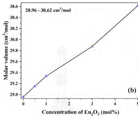
ภาพที่ 4.19 กราฟแสดงความสัมพันธ์ระหว่างปริมาตรเชิงโมลกับปริมาณความเข้มข้นของ \text{Eu}_2\text{O}_3
