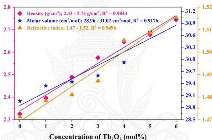
ภาพที่ 4.10 กราฟแสดงความสัมพันธ์ระหว่างความหนาแน่น ปริมาตรเชิงโมลและดัชนีหักเหของแก้วตัวอย่างกับปริมาณความเข้มข้นของ Tb_2O_3
