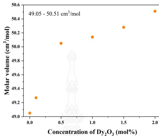
ภาพที่ 4.3 กราฟแสดงความสัมพันธ์ระหว่างปริมาตรเชิงโมลกับปริมาณความเข้มข้นของ \text{Dy}_2\text{O}_3
