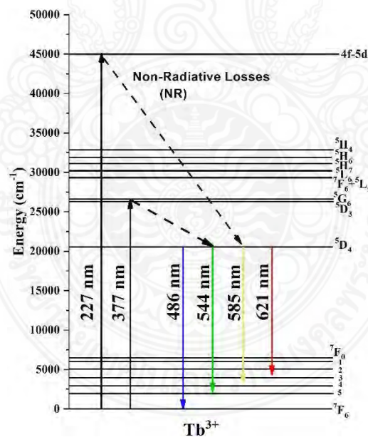
ภาพที่ 4.14 การเปลี่ยนแปลงระดับชั้นพลังงานของ \text{Tb}^{3+} เติมในแก้ว LNKB ตามสเปกตรัมการเปล่งแสง
