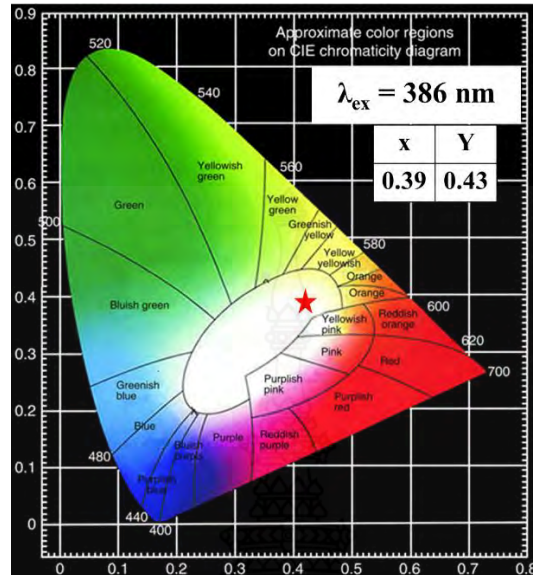
ภาพที่ 4.8 สีของการเปล่งแสงในระบบ CIE 1931 ของ Dy^{3+} เติมในแก้ว LNKDy
