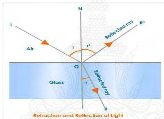
ภาพที่ 2.3 การหักเหและการสะท้อนของแสง ที่มา (วิฑิต วรรณเลิศลักษณ์, 2559: ออนไลน์)
