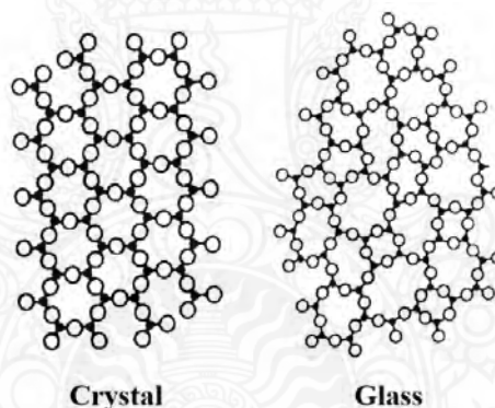
ภาพที่ 2.1 โครงสร้างของผลึกซิลิกาเกิดและแก้วซิลิกาเกิด ที่มา (Rao, 2002)
