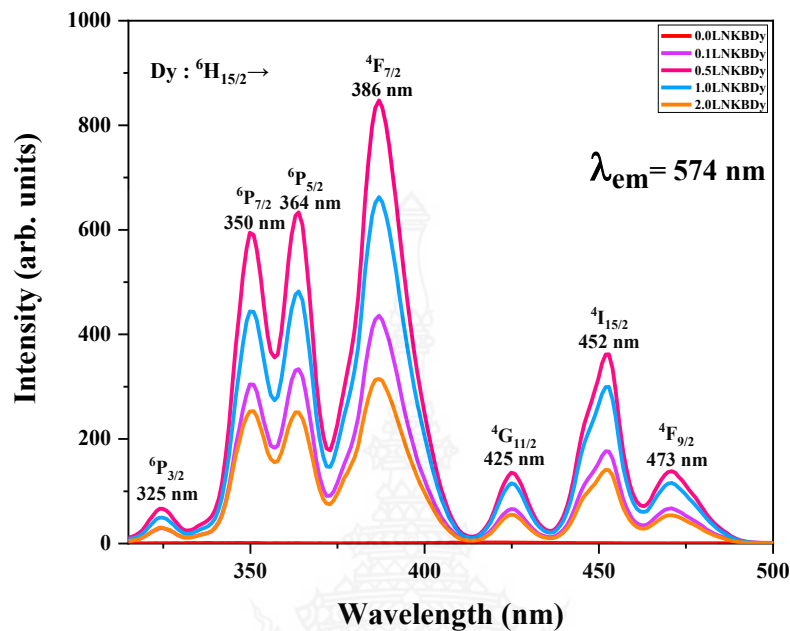
ภาพที่ 4.5 สเปกตรัมการกระตุ้นแสงของแก้วตัวอย่าง LNKB ที่เจือด้วย \text{Dy}_2\text{O}_3 ที่ความเข้มข้นต่าง ๆ
