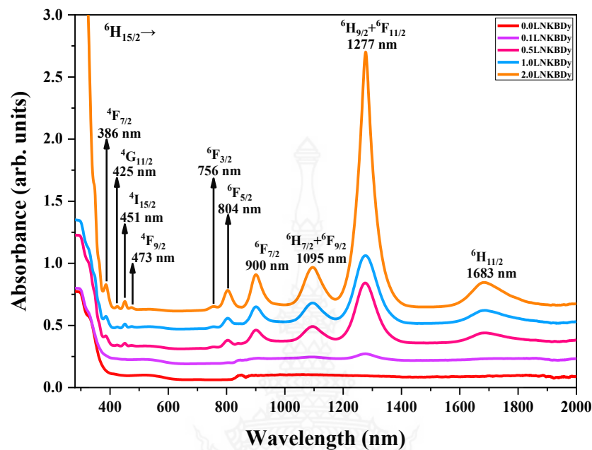
ภาพที่ 4.4 สเปกตรัมการดูดกลืนแสงของแก้วตัวอย่าง LNKB ที่เจือด้วย \text{Dy}_2\text{O}_3 ที่ความเข้มข้นต่าง ๆ
