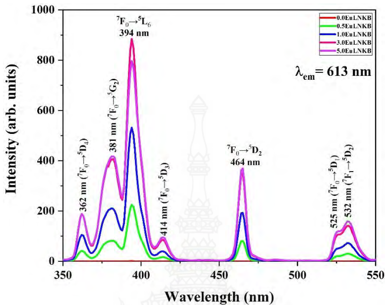
ภาพที่ 4.21 สเปกตรัมการกระตุ้นแสงของแก้วตัวอย่าง LNKb ที่เจือด้วย \text{Eu}_2\text{O}_3 ที่ความเข้มข้นต่าง ๆ
