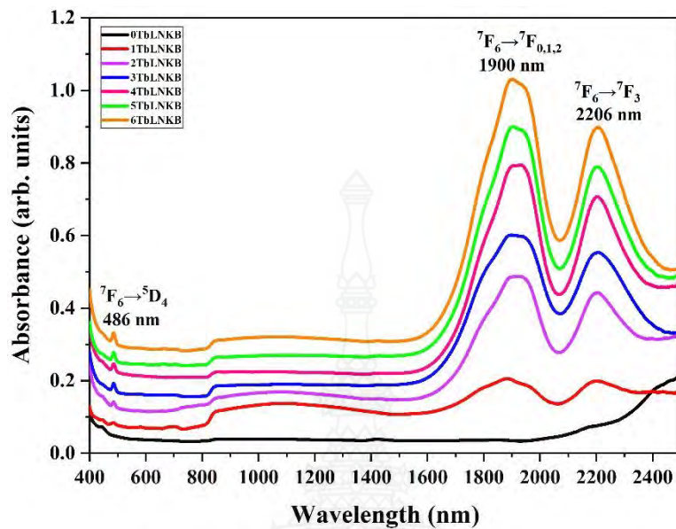
ภาพที่ 4.11 สเปกตรัมการดูดกลืนแสงของแก้วตัวอย่าง LNKB ที่เจือด้วย Tb_2O_3 ที่ความเข้มข้นต่าง ๆ
