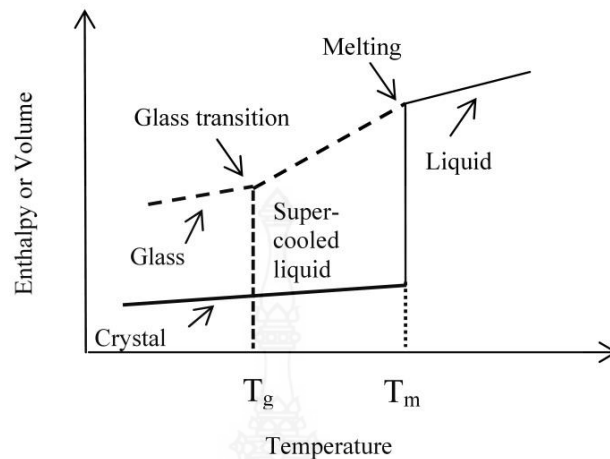
ภาพที่ 2.2 แผนภาพ V-T diagram
