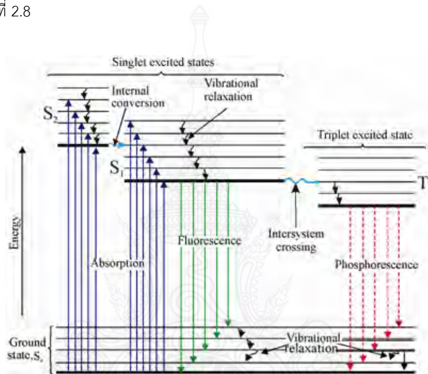
ภาพที่ 2.8 แผนภาพ Jablonski Diagram ที่มา (Bett, 2014: online)
