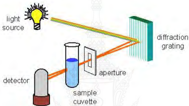
ภาพที่ 2.5 ส่วนประกอบของเครื่อง UV-Vis Spectrophotometer
